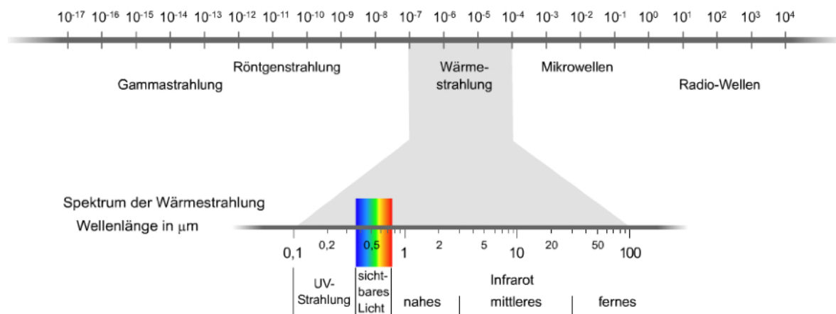
Bild 1.4: Wärmestrahlung im elektromagnetischen Spektrum
